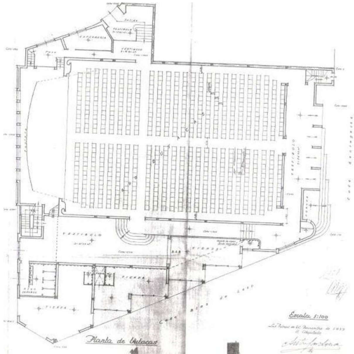
Plano del Cine Litoral
